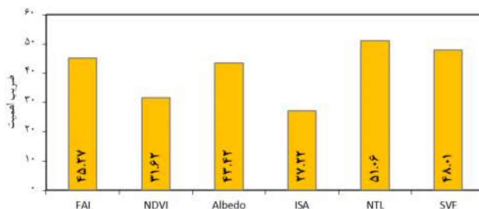
شکل (۳): نمودار اهمیت شاخص‌های مؤثر بر متوسط دمای سطح زمین
